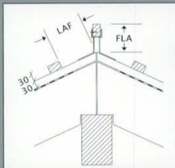
Balos oromszegély kialakítás félcseréppel*
