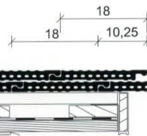
Jobbos oromszegély kialakítás félcseréppel*
