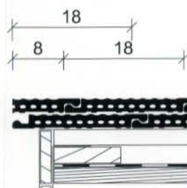
Balos oromszegély kialakítás félcseréppel*
